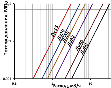
ПРИЛОЖЕНИЕ 2 Диаграмма потери давления
